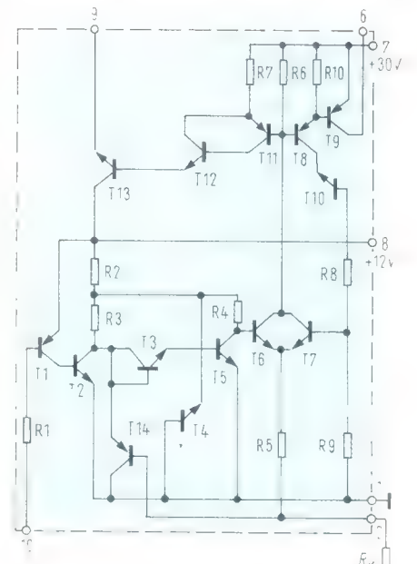
Bild 1. Aufbau einer der vier Stufen der IS SAS 560
