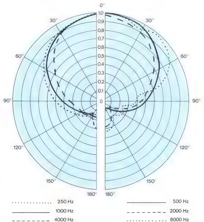
Bild 7. Richtdiagramm des Elektret-Mikrofones MKE 401
