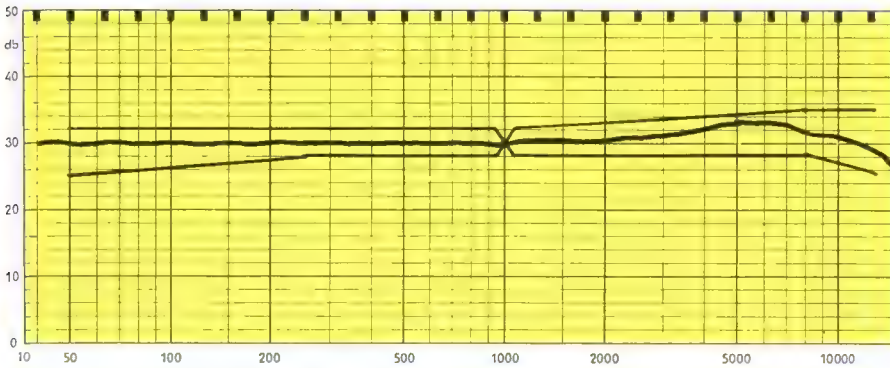
Bild 5. Leerlauf-Übertragungsmaß MKE 201
