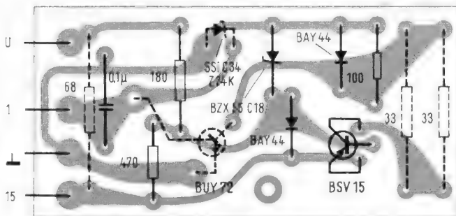
Bild 6. Platine und Bestückungsplan (die gestrichelten Bauteile sind auf dem Kühlkörper montiert)
