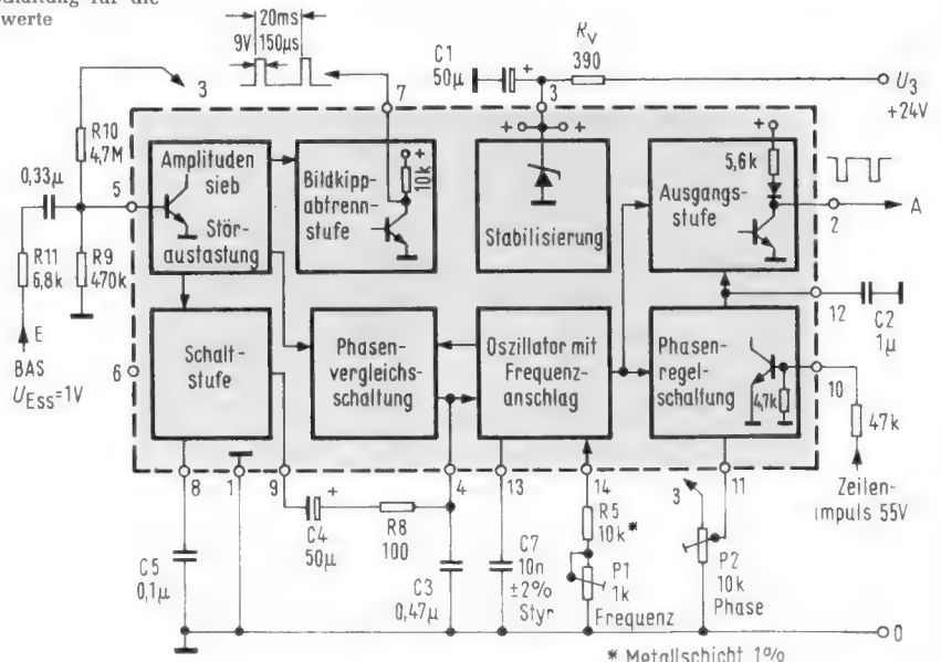
Bild 2. Blockschaltbild des TBA 940 und Meßschaltung für die Kennwerte
