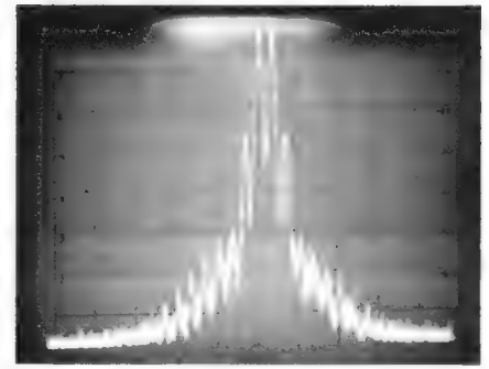
Bild 20. Darstellung des Intermodulationsverhaltens wie in Bild 19, jedoch mit einer Auflösung von 10 kHz/div. Das Grundrauschen stammt vom Analysator
