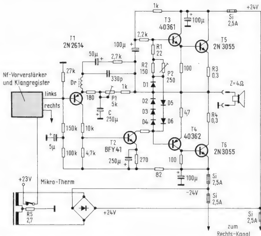
Schaltung einer Endstufe mit elektronischer Sicherung beim Steuergerät Hifi-Studio III E von Saba
