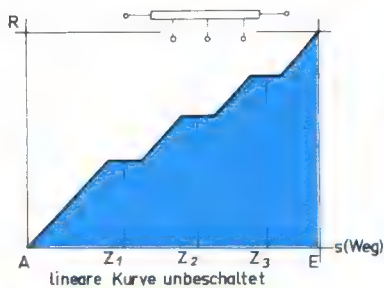
Bild 14. Lineare Kurve, unbeschaltet
