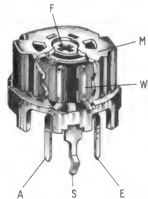
Bild 6. Aufbau eines Drahttrimmerwiderstandes. M = Isolierkörper; W = Widerstandselement mit Drahtwicklung und Anschlußbahnen A und E; S = Schleiferanschluß; F = Schleifeder mit Schraubendreherschlitz
