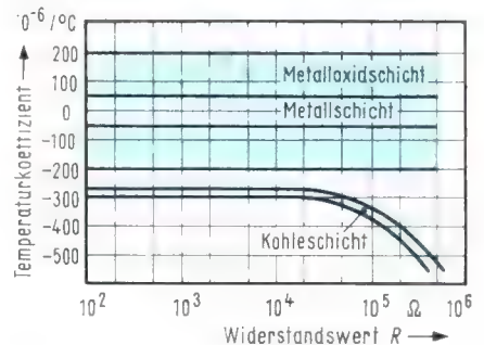
Bild 2. Abhängigkeit des Temperaturkoeffizienten vom Widerstandswert
