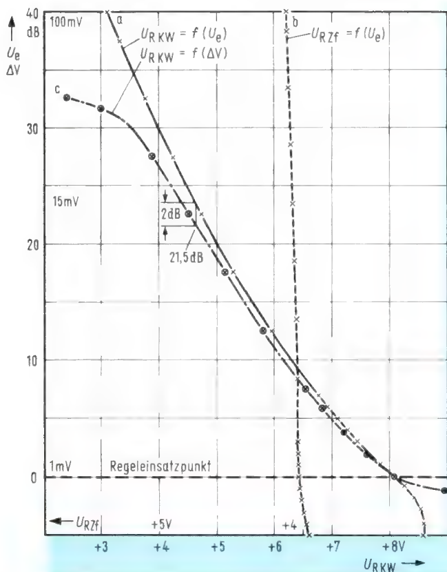
Bild 11. a = Tunerregelspannung im Empfänger für verschiedene Eingangsspannungen bei konstanter Ausgangsspannung; b = Zf-Regelspannung unter gleichen Bedingungen; c = für den Tuner allein gemessene Regelkurve
