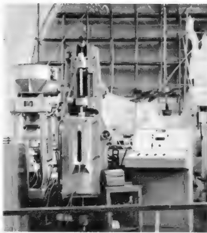
Bild 1. Einkristall-Ziehmaschine für Silizium
