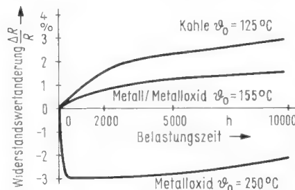
Bild 1. Widerstandswertänderung bei elektrischer Langzeitbelastung mit Gleichspannung
