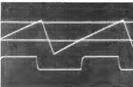
Bild 6. Schalten des Ausgangsimpulses
