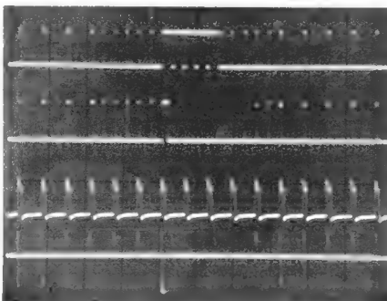
Bild 5. Impulsdiagramm der Phasenvergleichschaltung, von oben nach unten: BAS-Signal, BAS-Signal mit ausgetastetem Bildimpuls, Zeilenrückschlagimpulse am Anschluß 10, Regelstromimpulse
