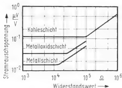
Bild 4. Vergleich der Mittelwerte des Stromrauschens der einzelnen Schichten
