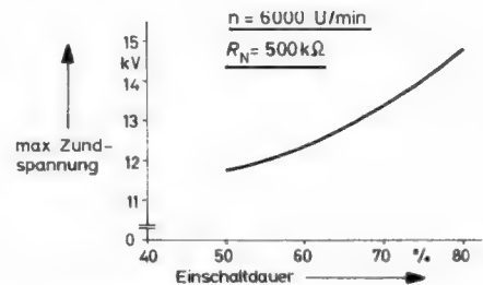
Bild 9. Transistor-Spuleneinschaltdauer
