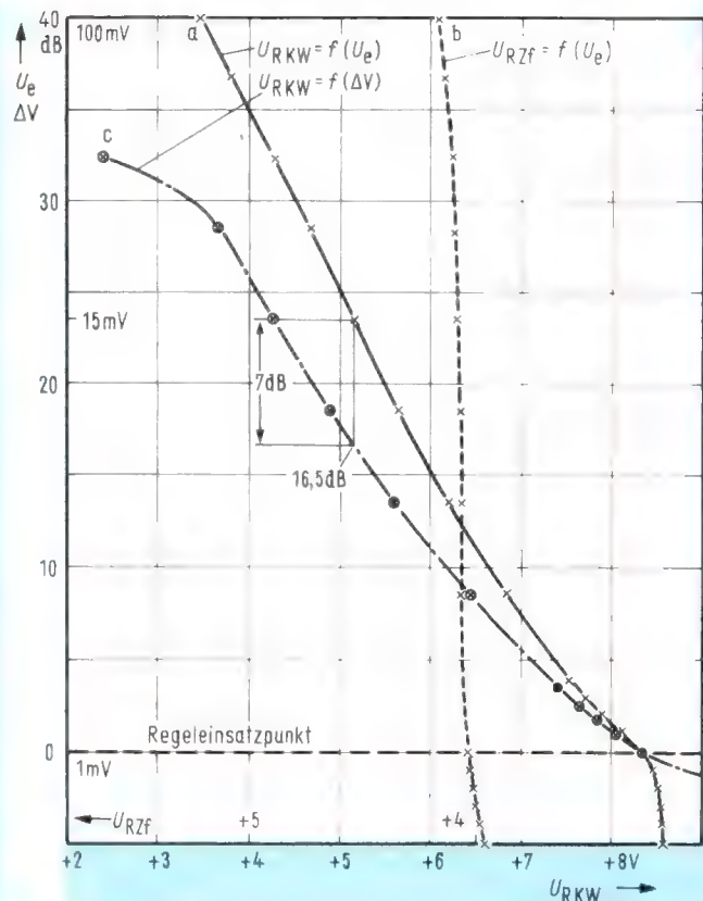
Bild 12. Die gleichen Kurven mit einem Regelverstärker erheblich geringerer Steilheit
