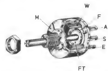
Bild 7. Aufbau eines Drahtdrehwiderstandes. M = Gehäuse mit Gewindebuchse und Wellenlagerung; W = Widerstandselement mit den Anschlüssen A und E; F = Schleifeder galvanisch mit Schleifring und Anschluß S verbunden; FT = Federträger
