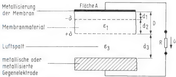
Bild 3. Elektret-Modell nach Sessler
