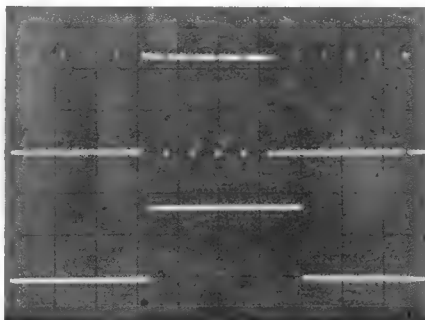
Bild 4. Integration der Bildimpulse: oben BAS-Signal, unten Bildimpuls am Anschluß 7
