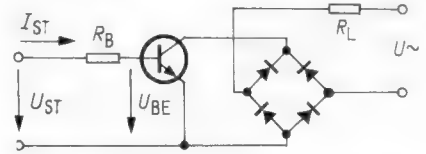
Einfacher Schalter für Wechselstromverbraucher
