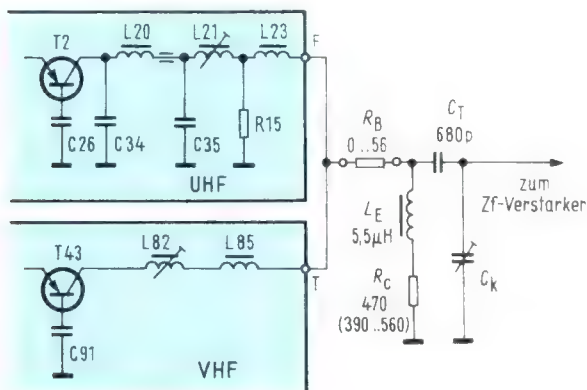
▲ Bild 4. Zf-Ausgang der Tuner UD 1 und VD 1
