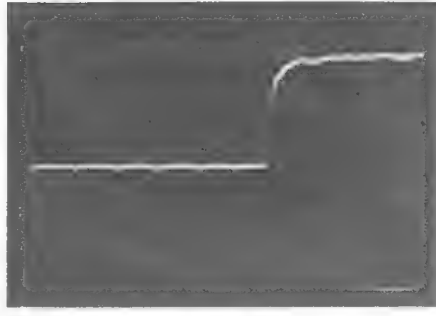
Bild 7b. Unterbrechung im Verteilernetz, Rechteckimpuls
