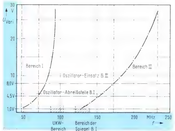
Bild 5. Verlauf der Abstimmspannung über der Frequenz
