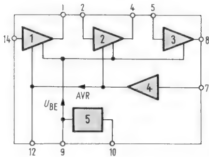
Bild 1. Blockschaltung des Zf-Verstärkerbausteins TBA 110 (Intermetall)
