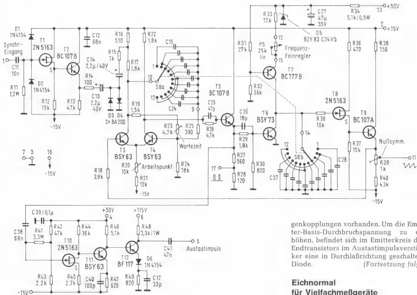
Bild 4. Kippteil mit Austastung
