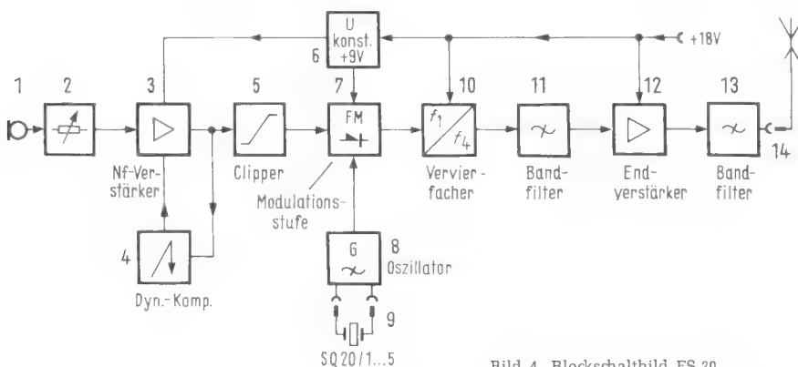
Bild 4. Blockschaltbild FS 20
