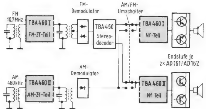
Bild 5. Stereo-Empfänger mit zwei Bausteinen TBA 460
