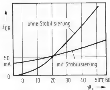
Bild 14. Ruhestrom einer Linear-Endstufe in Abhängigkeit von der Kühlkörpertemperatur ohne eine Stabilisierungsschaltung und mit der in Bild 13 gezeigten Stabilisierungsschaltung
