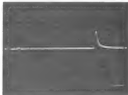
Bild 7e. Unterbrechung einer längeren Leitung, Impulsform Sinus (siehe Text)
