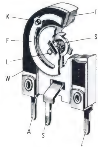
Bild 1. Aufbau eines Trimmerwiderstandes. T = Trägerplatte (Substrat); W = Widerstandselement mit den Anschlüssen A und E; F = Schleiffelder, die über der Krampe L mit dem Schleifring S in galvanischer Verbindung steht; K = Kohlekontakt und Metallkalotte
