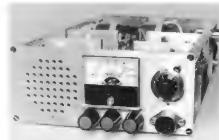
Bild 15. Vorderansicht eines mit eingebauter Batterie betriebenen 4-W-UKW-ESB-Transceivers (für BBT-Betrieb zugelassen), Gesamtgewicht = 1,95 kg
