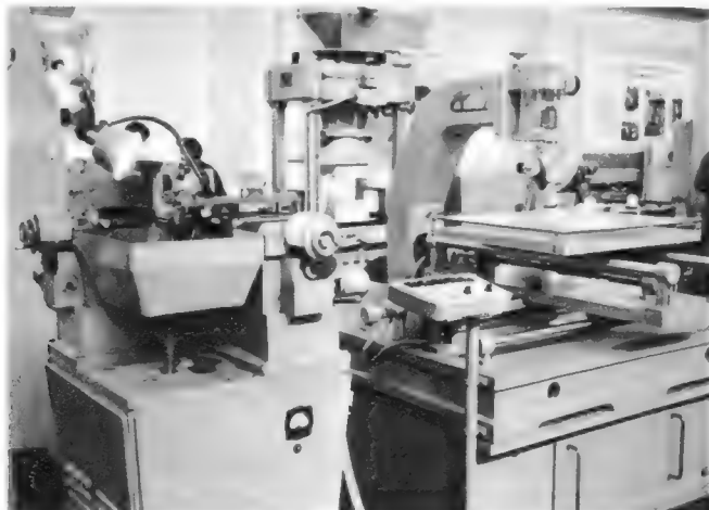
Bild 2. Funkenerosionsfräser (links), daneben die zugehörige Steueranlage mit Lichtpunktabtastung der Zeichnungsvorlage. Der Maßstab 30 : 1 war fixiert und konnte nicht verändert werden (Aufnahmen: Groll)
