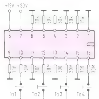
Bild 2. Meßschaltung für die in Tabelle 1 aufgeführten Daten
