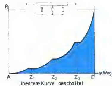
Bild 15. Lineare Kurve, beschaltet
