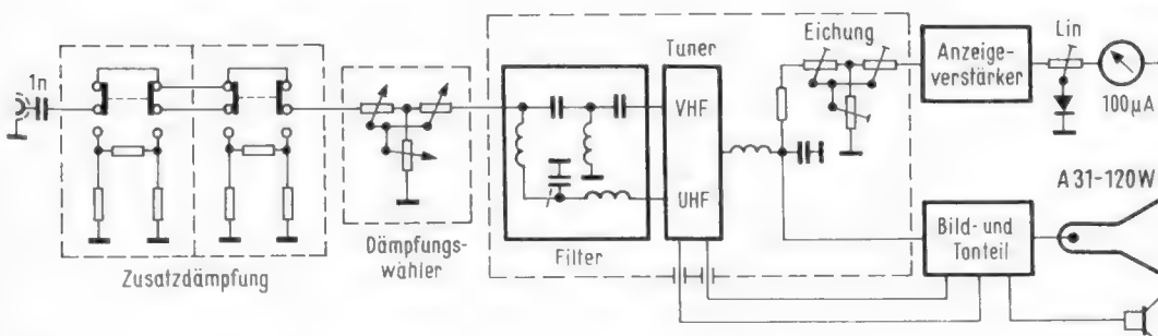
▲ Bild 4. Hochfrequenz-Millivoltmeter MUK 11
