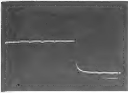
Bild 7a. Kurzschluß im Verteilernetz, Impulsform Rechteck
