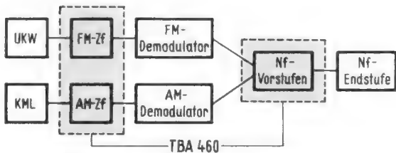
Bild 4. Im Baustein TBA 460 integrierte Stufen
