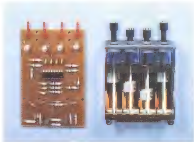
Bild 2. Ansicht eines Labormusters einer Vierer-Abstimmereinheit
