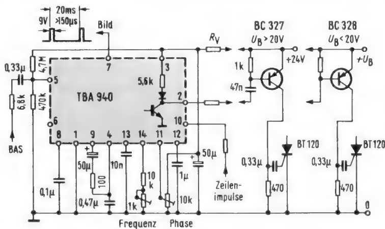
Bild 10. Ansteuerung einer Thyristor-Endstufe
