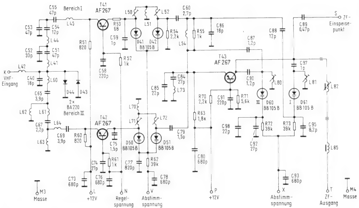
Bild 3. Schaltbild des VHF-Tuners 12 ET 5732/02 (VD 1)
