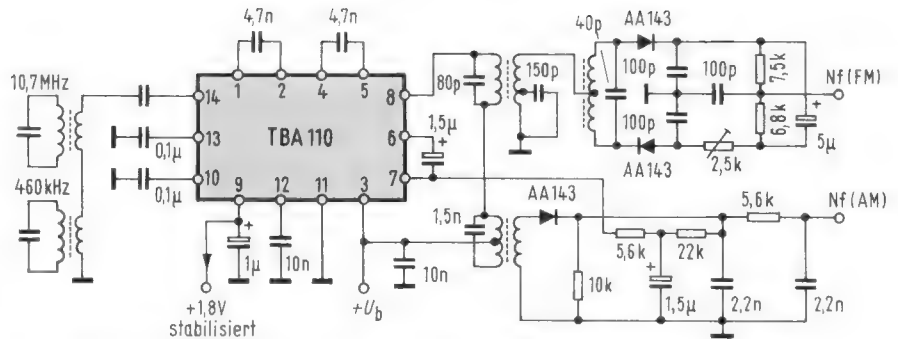
Bild 2. Anwendungsbeispiel für die integrierte Schaltung TBA 110
