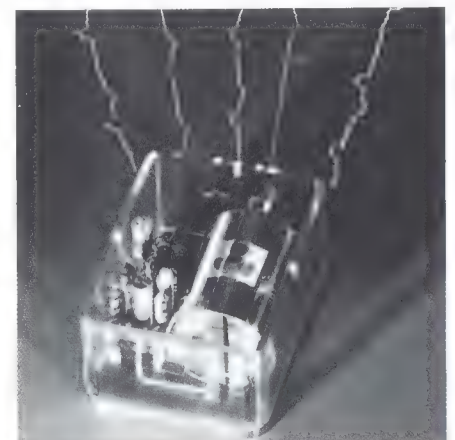
Labormodell des ersten deutschen Herzschrittmachers mit atomarer Energiequelle. Lebensdauer mindestens zehn Jahre
