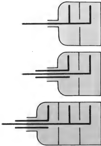
◀ Bild 2. Ausführungsformen von Schicht- bzw. Massedrehwiderständen. Oben: Tandem; Mitte: Doppeldrehwiderstand; Unten: Tandem-Doppeldrehwiderstand
