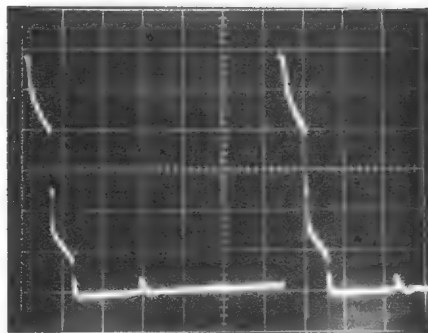
Bild 9. Impulse am Gate eines Thyristors
