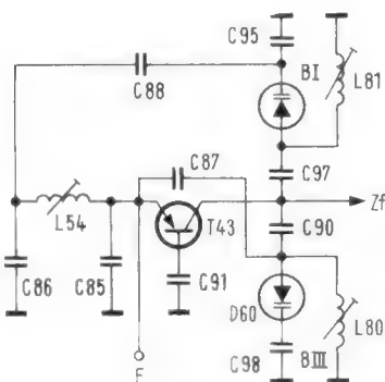
Bild 7. Selbstschwingende Mischstufe (Ausschnitt aus Bild 3)
