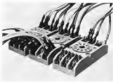
Bild 4. Stecksokkel mit AMP-Anschluß (Elesta)
