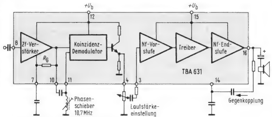
Bild 8. Blockschaltung des TBA 631 (SGS)
