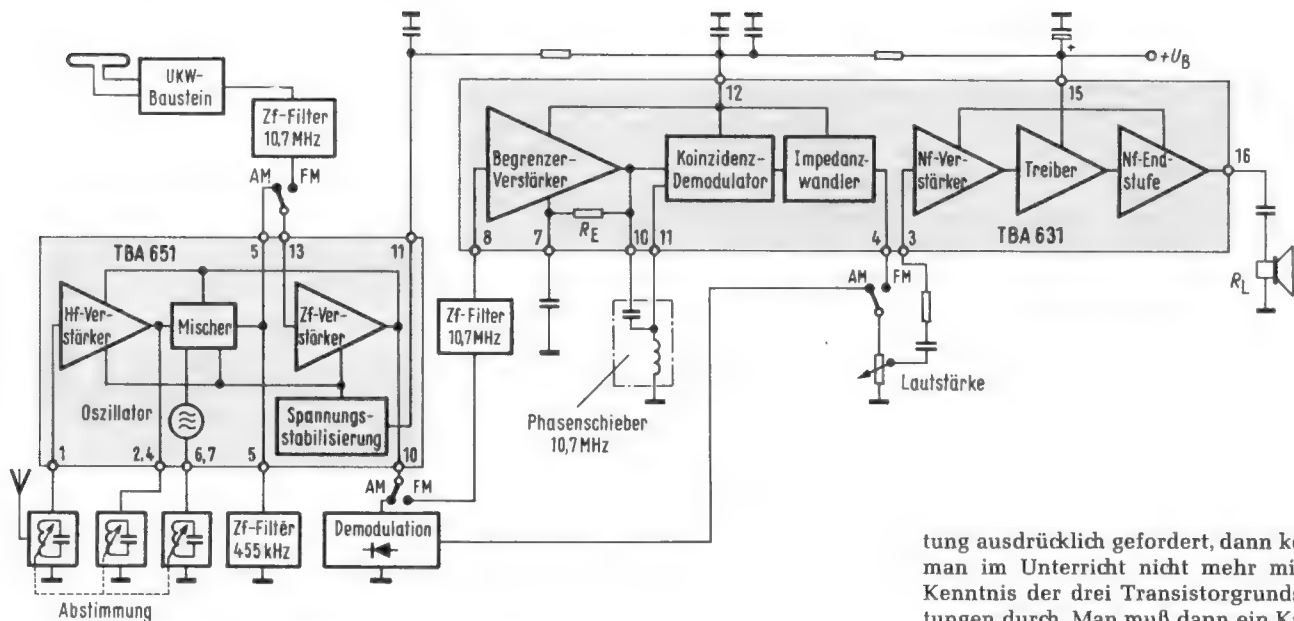
Bild 9. AM-FM-Empfänger mit zwei integrierten Schaltungen
