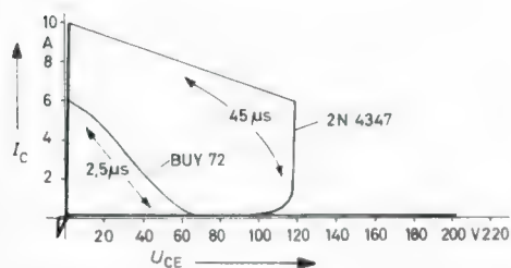
Bild 1. Transistorbelastung während der Abschaltung
