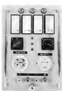
Drehstrom-Einschub 3x 380 V/10 A
