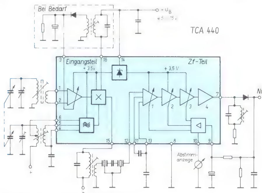
Blockschaltung des integrierten AM-Empfängers
