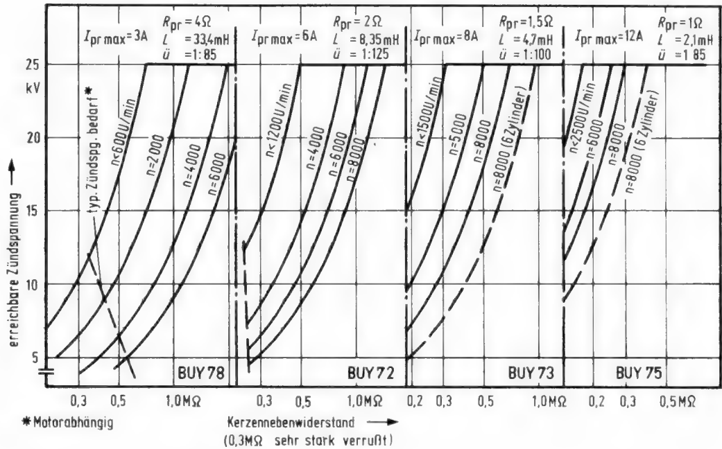
Bild 7. Zündspulen für Vierzylindermotoren. Spulenergie = maximal 150 mWs
