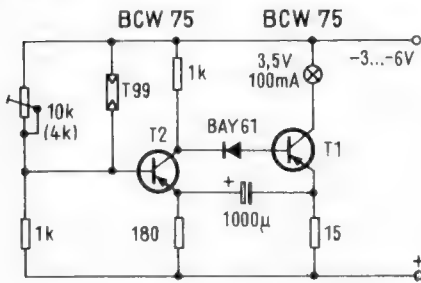
Schaltung des Dämmerungsblinkers
