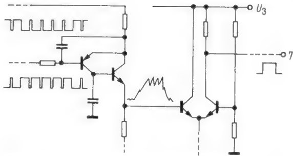
Bild 3. Prinzipschaltung der Bildimpuls-Integration
