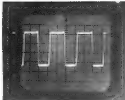
Bild 15. Das 1-MHz-Signal des Generators (horizontal 1/3 µs/Einh., vertikal 1 V/Einh.). Die Bandbreite des verwendeten Oszillografen beträgt etwa 10 MHz
