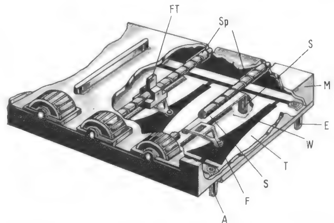
Bild 5. Schicht-Spindelwiderstand in einem Abstimmaggregat. M = Isoliergehäuse; T = Trägerplatte mit Widerstandsbahn W und Anschlußbahnen A und E; SP-Leitspindel; FT = Federträger mit Schleiffeder F; S = Schleiferanschluß
