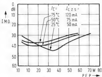
Bild 12. Intermodulationsverzerrungen dritter Ordnung ( d_3 ) als Funktion der Spitzenleistung (PEP) mit der Gehäusetemperatur ( T_c ) und dem entsprechenden Kollektorruhestrom I_{CzS} als Parameter
