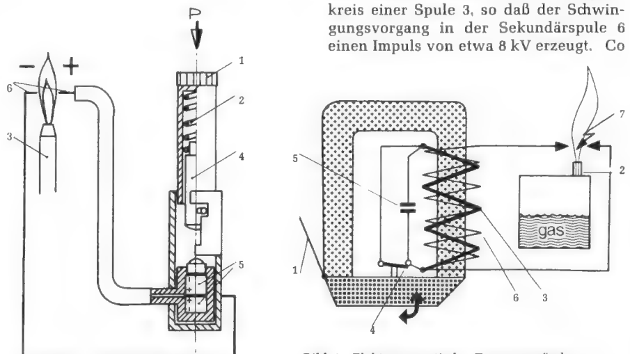
Bild 1. Prinzip eines Taschenfeuerzeuges mit piezokeramischer Zündung (Werkzeichnung: Consul)
