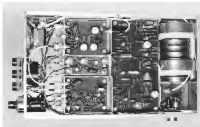
Bild 17. Blick in das geöffnete Gerät von der Empfängerseite her. Man erkennt neben dem Nickel-Cadmium-Akkumulator das für die Spiegelselektion des Empfängers und Nebenwellenabschwächung des Senders vorgesehene Helix-Bandfilter
