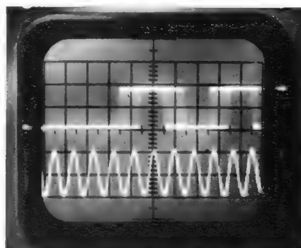
Bild 17 und 18. Bei 100 kHz sind die Impulsflanken um 10 % „verwackelt“, bei 250 kHz sogar um 25 %. Mit dem Potentiometer P läßt sich der erste Impuls über den ganzen Bildschirm verschieben
