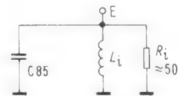
Bild 9. Ersatzbild für die Schaltung in Bereich III
