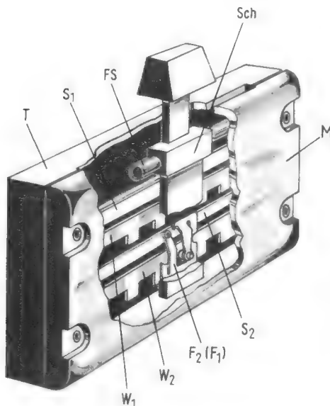
Bild 4. Aufbau eines Schichtschiebewiderstandes. T = Trägerplatte mit parallel angeordneten Widerstandselementen W 1 und W 2; S 1 und S 2 = die beiden zugeordneten Schleiferbahnen; Sch = Schieber, der in einem metallischen Ober teil M auf einer Führungsschiene FS gelagert ist; F 1 /F 2 = Schleiffedern, die die galvanische Verbindung zwischen Widerstandselementen und Schleiferbahnen S 1,2 herstellen
