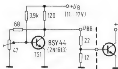
Bild 13. Stromlaufplan einer einfachen Temperaturstabilisierungsschaltung für die Basisvorspannung U_{BB} von transistorisierten Linear-Endstufen
