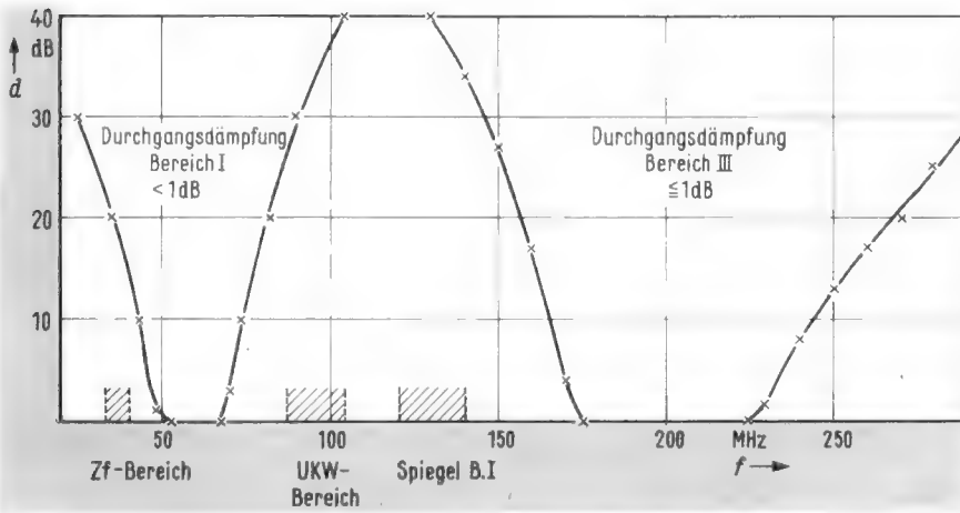
Bild 6. Dämpfungsgang der Eingangsfilter
