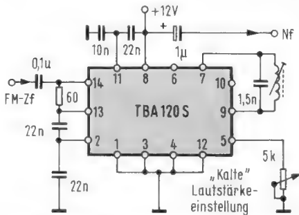
Bild 3. Baustein TBA 120 für einen FM-Zf-Verstärker mit Koinzidenzdemodulator (Siemens)
