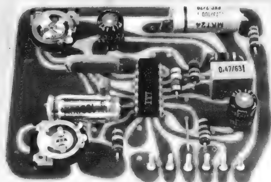
Bild 8. Bestückte Platine mit der integrierten Schaltung TBA 950
