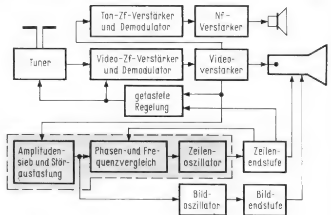
Bild 1. Blockschaltbild eines Schwarzweiß-Fernsehempfängers
