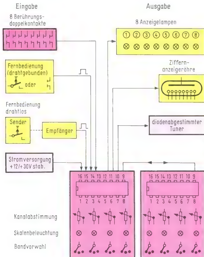
Bild 3. Blockschaltbild einer 8fach-Sensoranlage mit Erweiterungsmöglichkeiten
