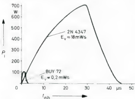
Bild 2. Abschaltverlustleistung am Transistor
