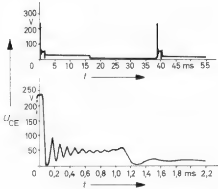
◀ Bild 4. Spannungsverlauf am Transistor
