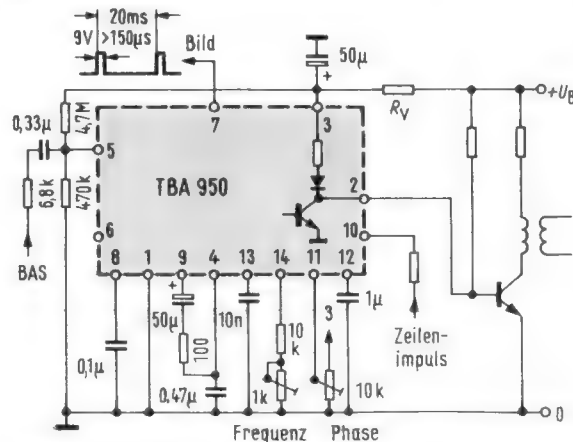
Bild 11. Ansteuerung einer Transistor-Endstufe
