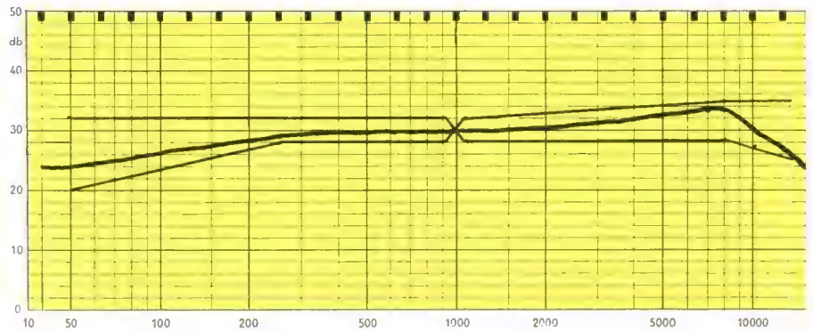
Bild 6. Leerlauf-Übertragungsmaß MKE 401
