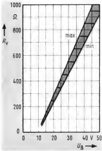
Bild 7. Diagramm zur Ermittlung des Vorwiderstandes R_V
