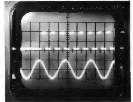
Bild 16. Aufgrund des eingblendeten 1000-Hz-Signals kann die Frequenz des Sinussignals bestimmt werden: 360 Hz. Daß die Signalform der Impulsreihe gegenüber Bild 14 etwas verzerrt ist, rührt vom verwendeten Zweikanalzusatz her
