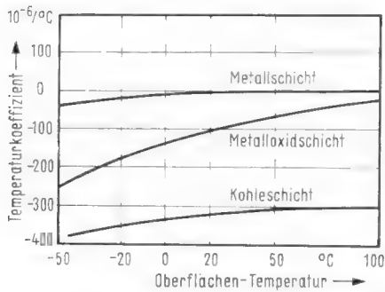
◀ Bild 3. Verlauf der Temperaturkoeffizienten der drei Schichtarten als Funktion der Temperatur
