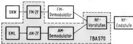
Bild 6. Integrierte Schaltungsstufen im Baustein TBA 570
