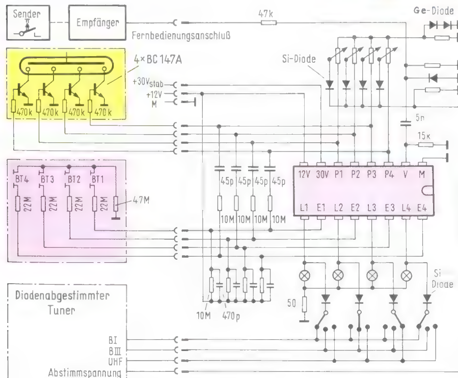
Bild 1. Schaltbild einer Sensor-Vierereinheit mit IS
