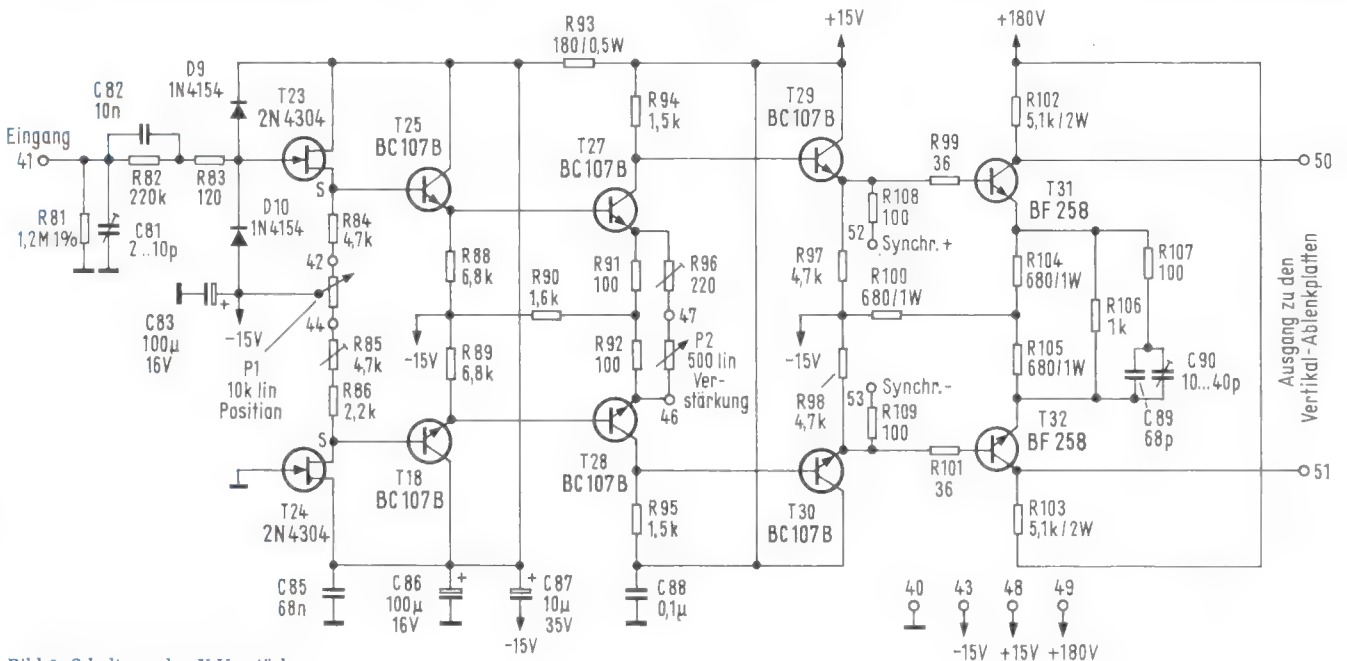
Bild 3. Schaltung des Y-Verstärkers
