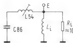
Bild 8. Ersatzbild für die Schaltung in Bereich I
