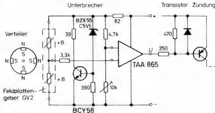
Bild 8. Kontaktloser Unterbrecher mit dem Feldplattengeber GV 2
