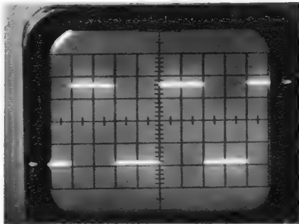
Bild 14. Das 1000-Hz-Signal des Generators (horizontal 250 µs/Einh., vertikal 1 V/Einh.)
